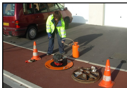
Test à la fumée à DOUAI
